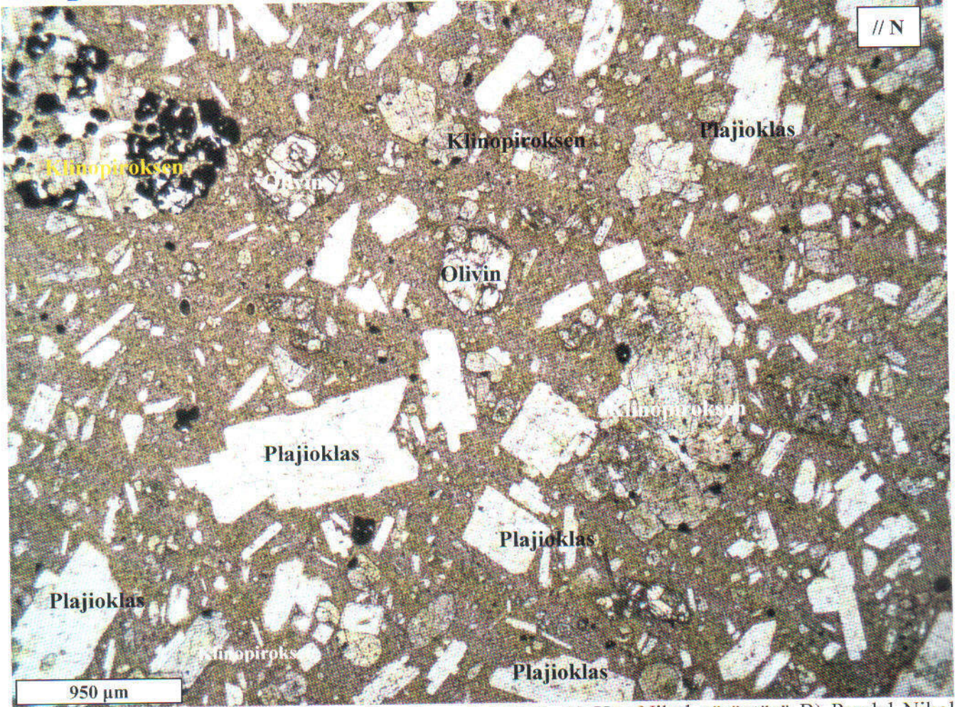
Şekil 1. Bazalt örneğinin polarizan mikroskop görüntüsü. A) Haç Nikol görüntüsü B) Paralel Nikol görüntüsü
